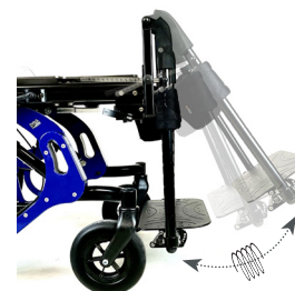
Reposapiernas elevables con amortiguación Free-Shock con opción de bloqueo
