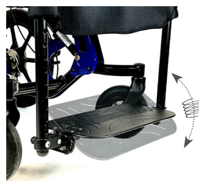
Plataforma reposapiés con movimiento de flexión dorsal/plantar Free-Shock
