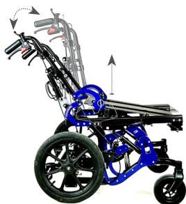
Sistema de respaldo-asiento dinámico Free-Shock
